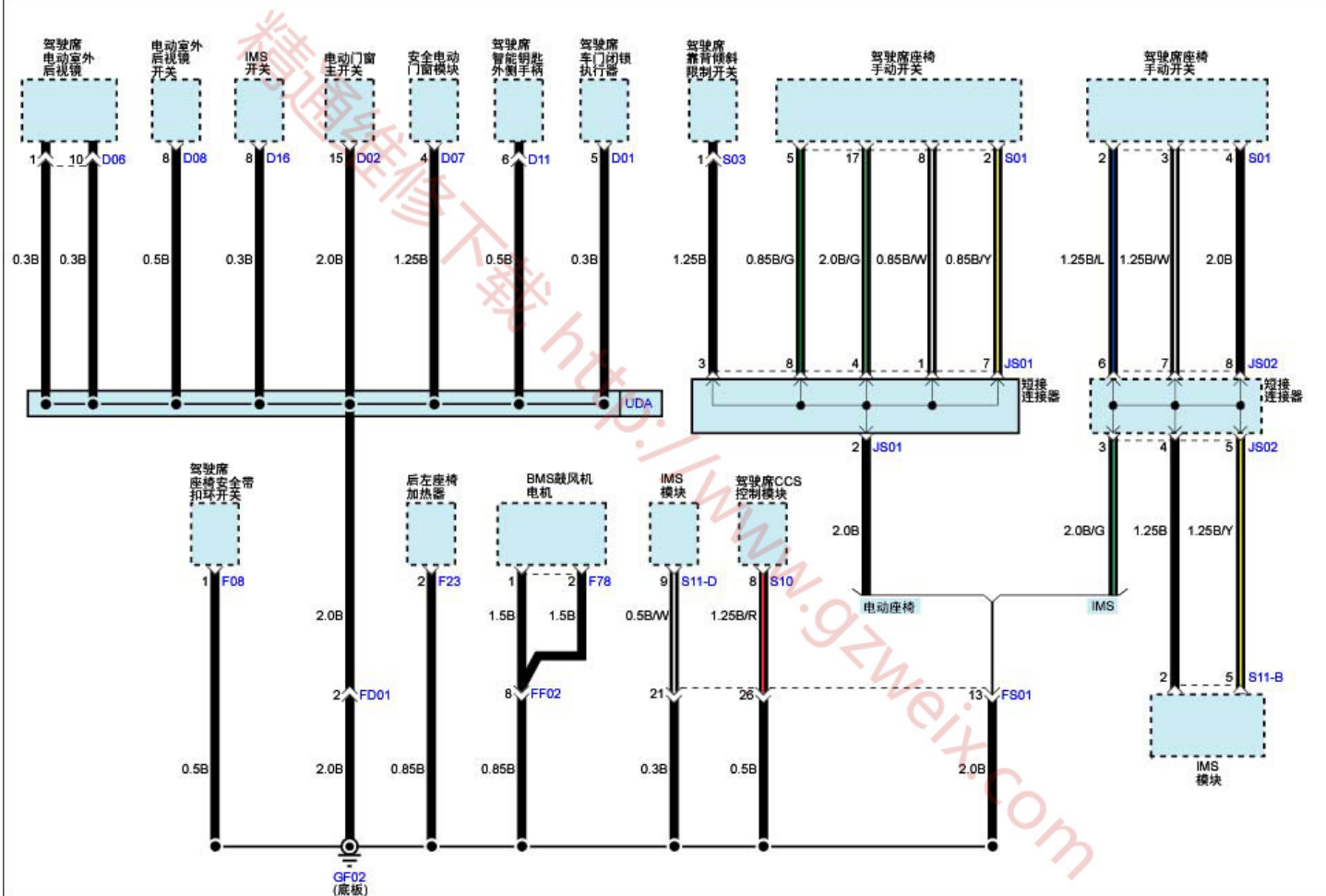
搭铁分布(5)
